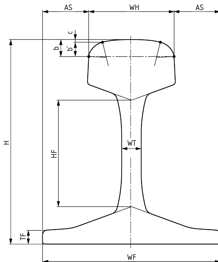
Rysunek 1 Odniesienia do tolerancji wymiarowych (wg Tablicy 7)
