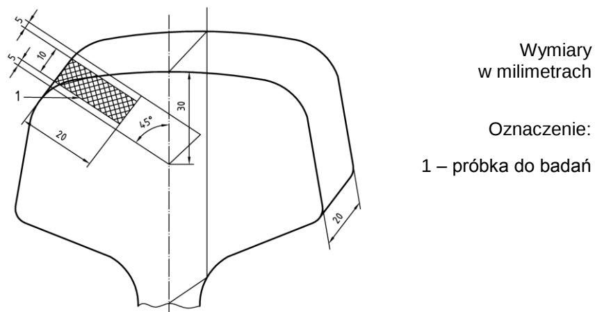
Rys. 6 Miejsce pobierania próbki w głowce szyny do badania czystości tlenkowej
